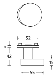
Knopf zyl. versetzt
