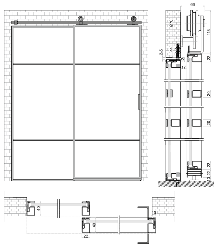
DE | Einzelschiebetür mit seitlichem Fix-Element EN | Single Sliding Door with Side Fixed Element
