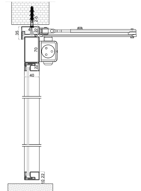
DE | Option mit oberem Türschließer EN | Option with Overhead Door Closer
