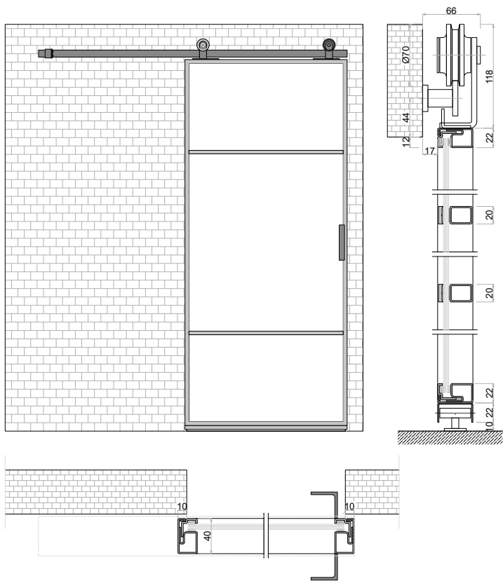
DE | Einzelschiebetür EN | Single Sliding Door
