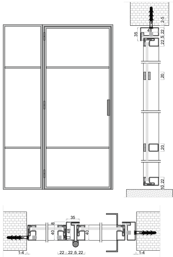
DE | Einzeltür mit seitlichem Fix-Element EN | Single Door with Side Fixed Element
