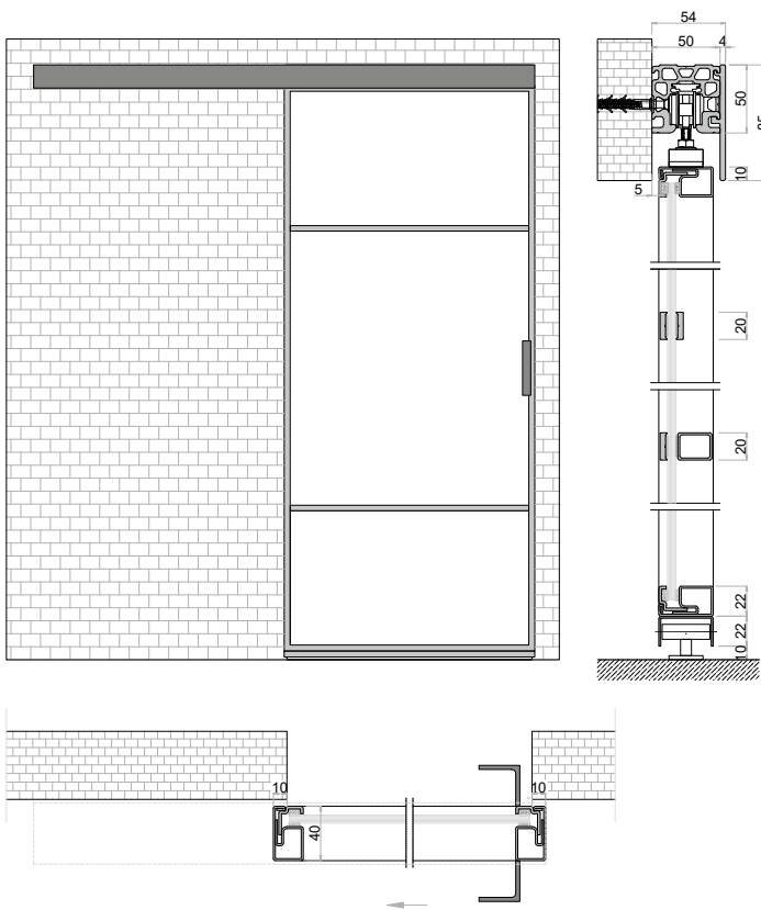
DE | Einzelschiebetür mit Wandmontage EN | Single Sliding Door with Wall Mounting
