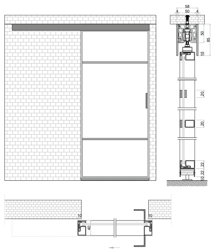
DE | Einzelschiebetür mit Deckenmontage EN | Single Sliding Door with Ceiling Mounting
