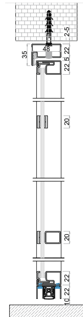
DE | Option mit absenkbarer Bodendichtung EN | Option with Drop-Down Floor Seal
