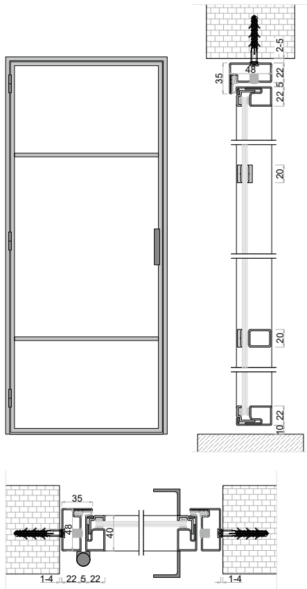
DE | Einzeltür EN | Single Door
