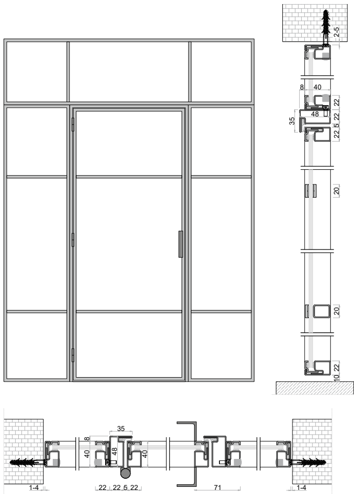
DE | Einzeltür mit zwei seitlichen Fix-Elementen und Oberlicht EN | Single Door with Two Side Fixed Elements and Top Transom
