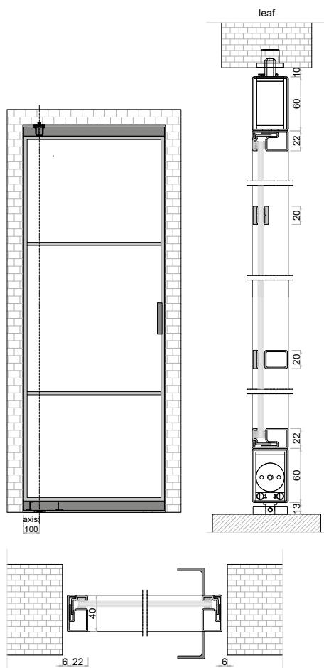
DE | Einzeltür Pivot EN | Single Pivot Door
