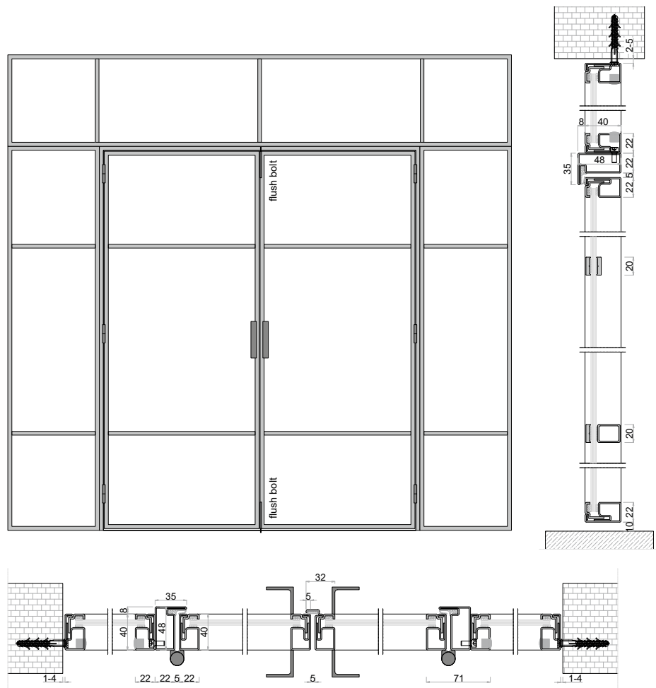
DE | Doppeltür mit zwei seitlichen Fix-Elementen und Oberlicht EN | Double Door with Two Side Fixed Elements and Top Transom
