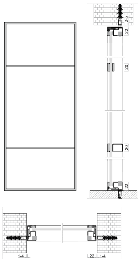
DE | Einzelnes Fix-Element EN | Single Fixed Element
