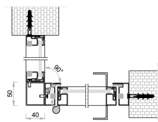
DE | Verbindung von Fix-Element und Tür mit Eckpfosten EN | Connection of Fixed Element and Door with Corner Post
