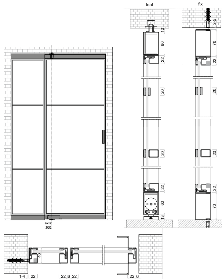
DE | Einzeltür Pivot mit seitlichem Fix-Element EN | Single Pivot Door with Side Fixed Element
