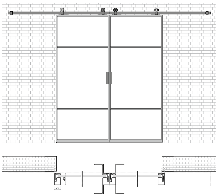
DE | Doppelschiebetür EN | Double Sliding Door
