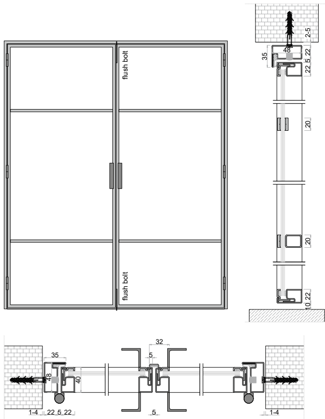
DE | Doppeltür EN | Double Door
