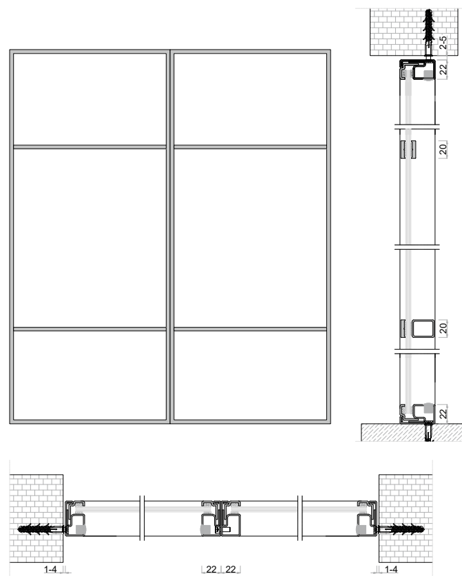
DE | Doppeltes Fix-Element EN | Double Fixed Element
