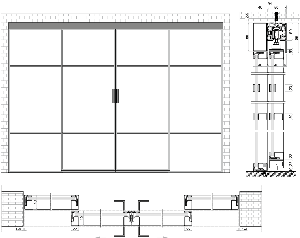
DE | Doppelschiebetür mit zwei seitlichen Fix-Elementen EN | Double Sliding Door with Two Side Fixed Elements
