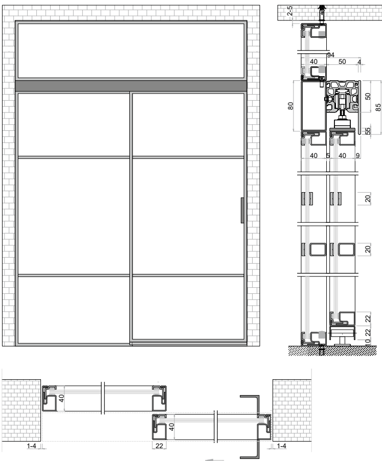
DE | Doppelschiebetür mit festem Seitenteil (Fix) EN | Double Sliding Door with Fixed Side Panel
